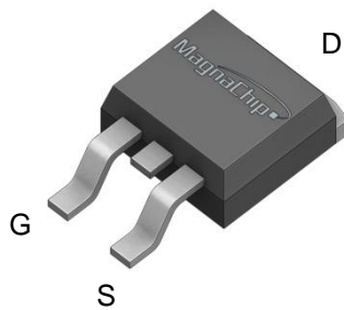
TO-263
